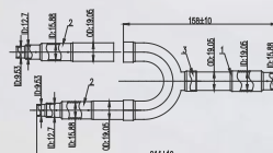
Rozdzielacze RVF- RDIX17
