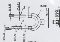
Rozdzielacz do cieczy
